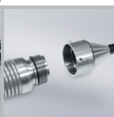
Adattatore intercambiabile per la sostituzione della testina di ripresa
